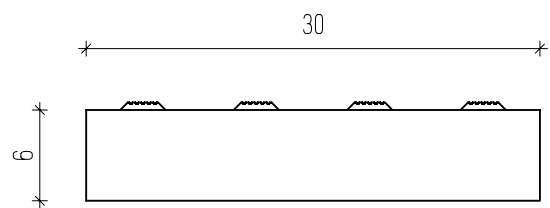
Elölnézet
