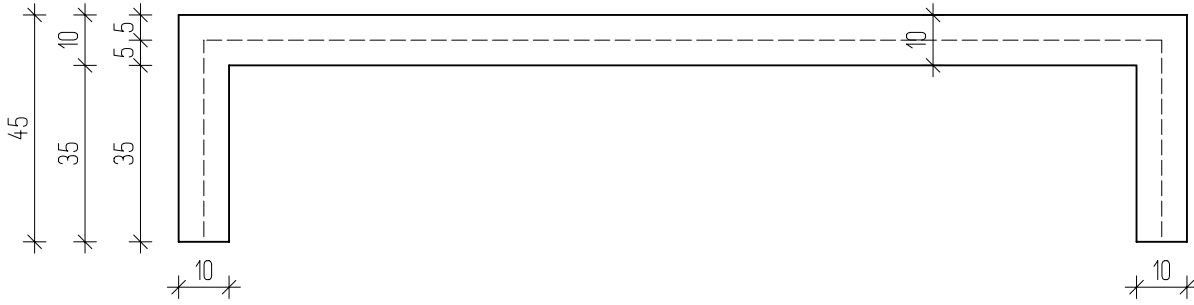
Felülnézet
