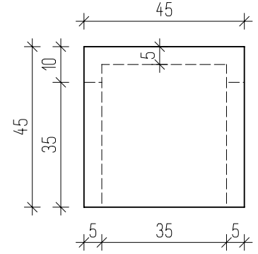
Oldalnézet
