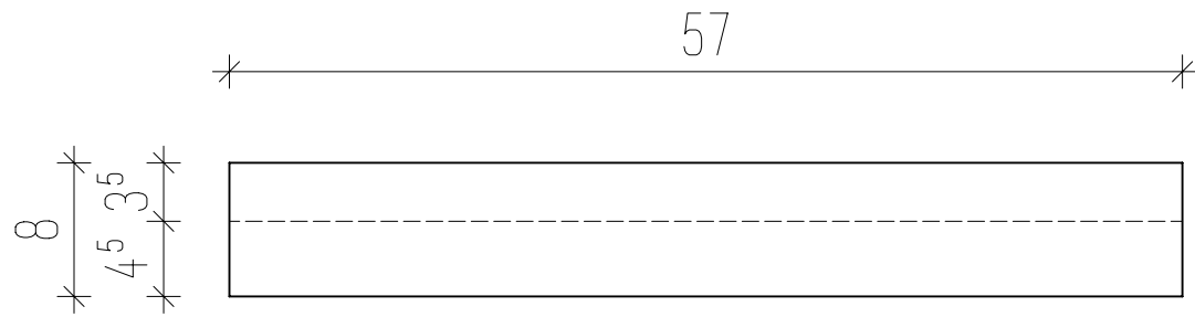
Felülnézet
