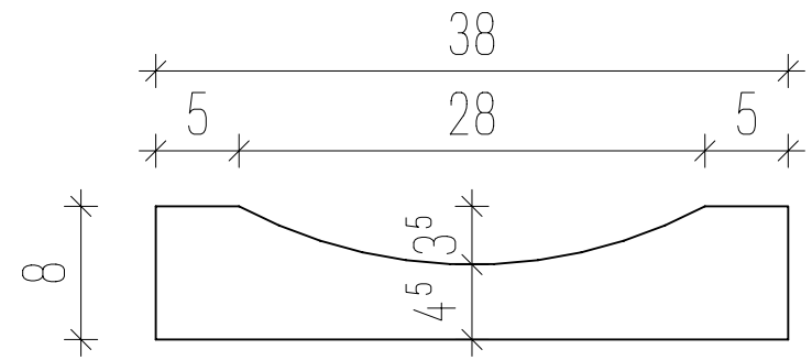
Oldalnézet
